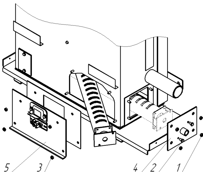
Рисунок 2а. Демонтаж основной горелки:
