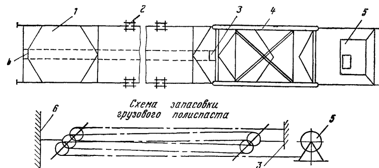
Рис. 25. Инвентарный накаточный путь для монтажа водогрейного котла методом надвижки.
