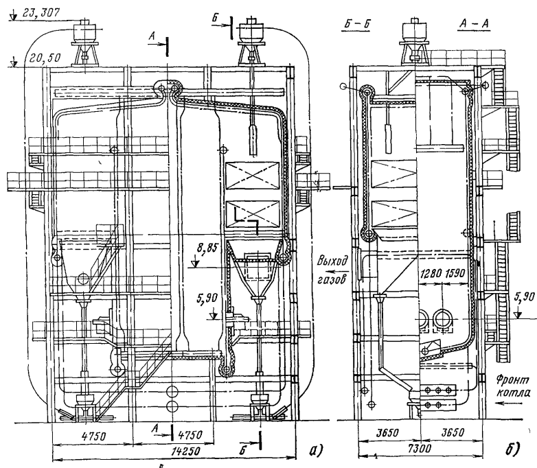
Рис. 2. Общий вид газомазутного водогрейного Т-образного котла KB-ГМ-180 теплопроизводительностью 210 МВт.
