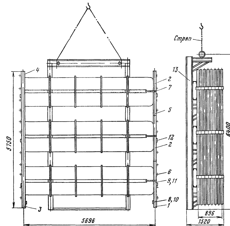
Рис. 20 Монтажный блок конвективной части котла КВ-ГМ-100.
