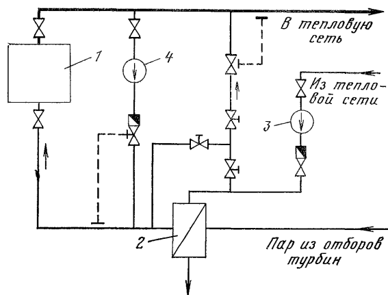
Рис. 1. Схема установки пиковых котлов на ТЭЦ. 1 — пиковый котел; 2 — подогреватель; 3 — сетевой насос; 4 — рециркуляционный насос.
