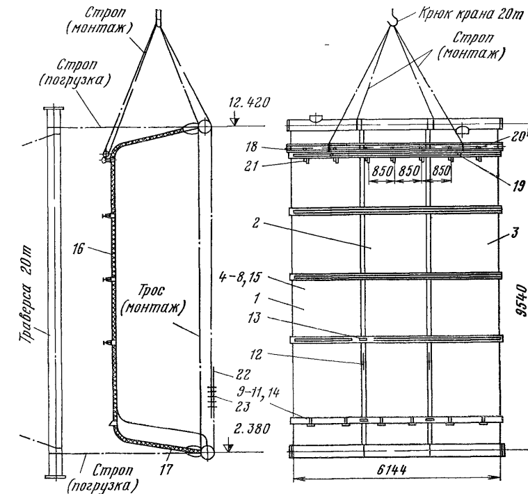
Рис. 18. Монтажный блок левого бокового экрана котла КВ-ГМ-100.
