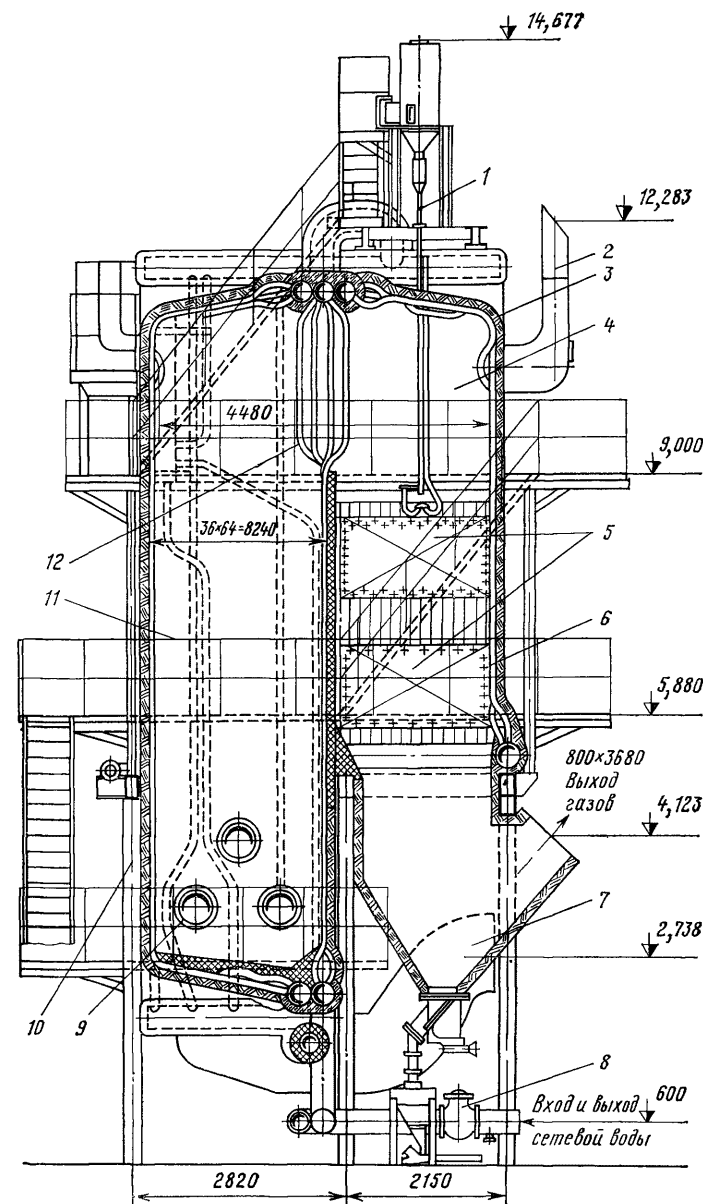
Рис. 10. Котел ПТВМ-30М-4.
