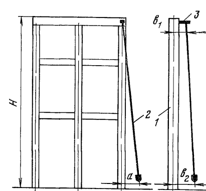
Рис. 15 Проверка вертикальности блока каркаса по отвесу
